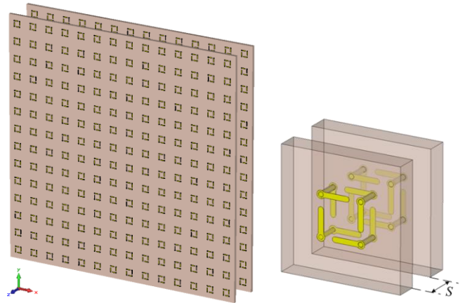
Fig. 2. Doble lámina con detalle de la doble celda unidad.
